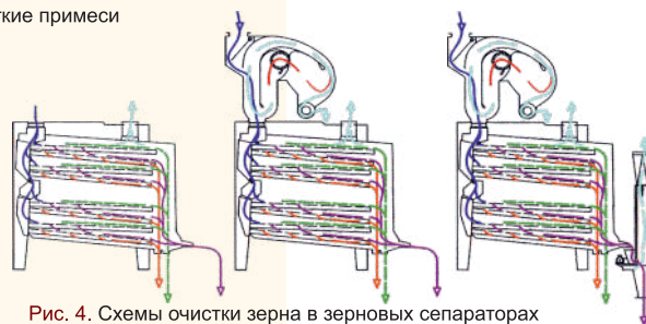
Рис. 4. Схемы очистки зерна в зерновых сепараторах «ГОРИЗОНТ-К-250», «ГОРИЗОНТ-К-300» и «ГОРИЗОНТ-К-400»
